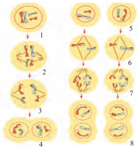
Рис.32. Мейоз.
