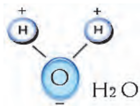
Рис.3. Молекула воды
