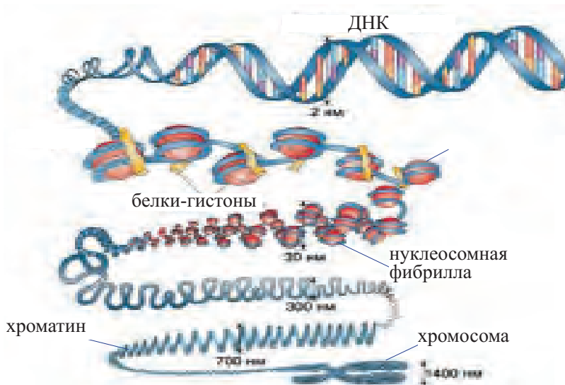
Рис.28. Структура хромосомы.
