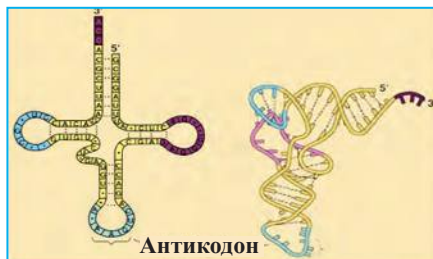
Рис.18. т-РНК.
