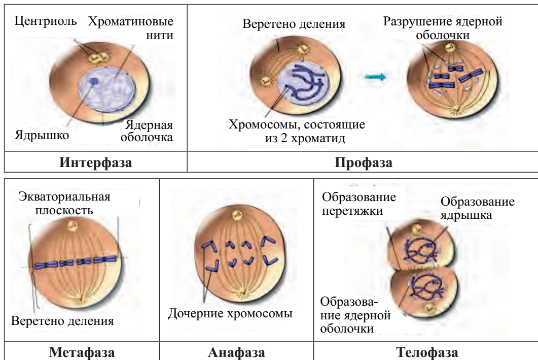
Рис.30. Этапы митоза.
